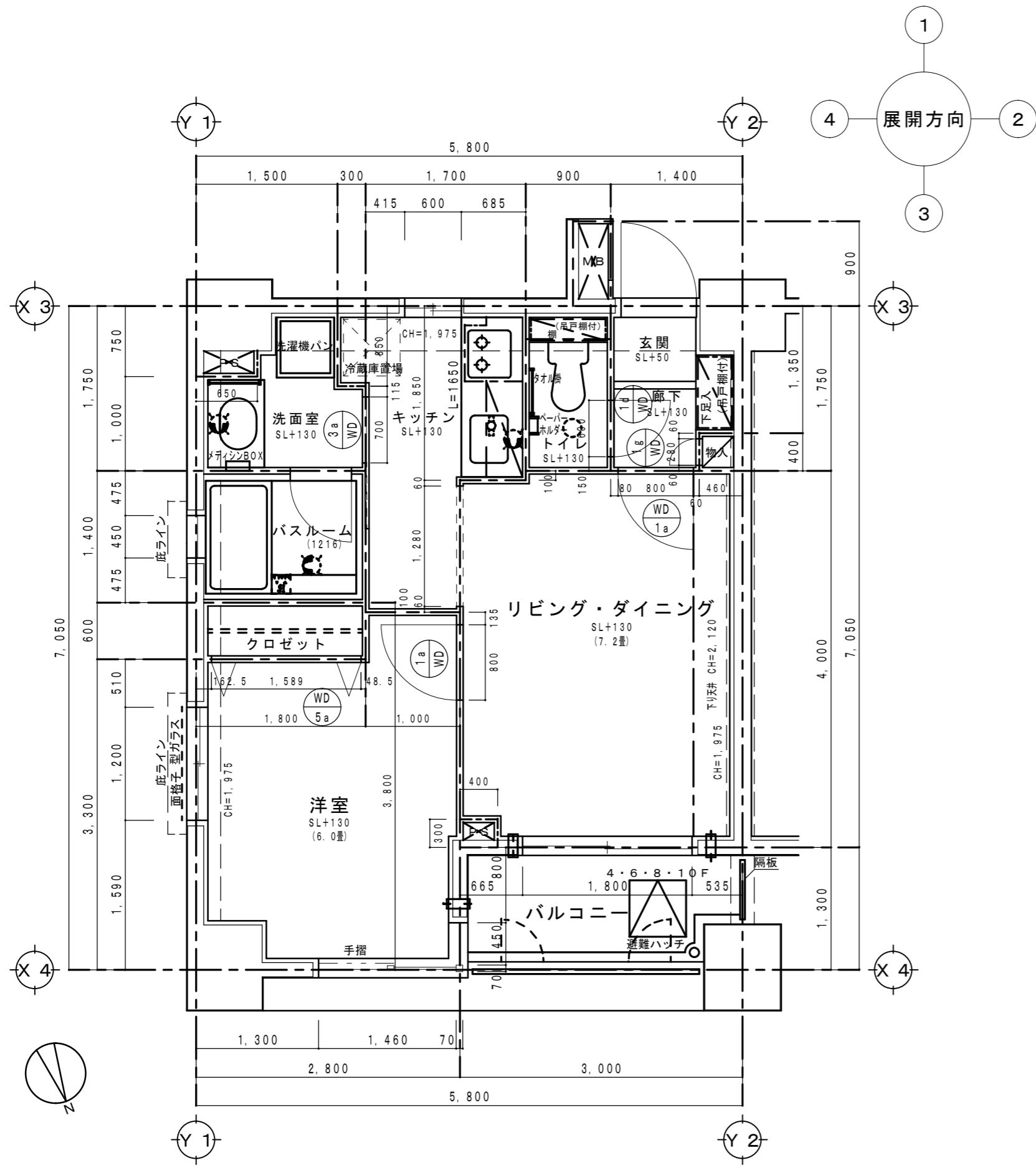
B1タイプ 平面詳細図 S=1:50
