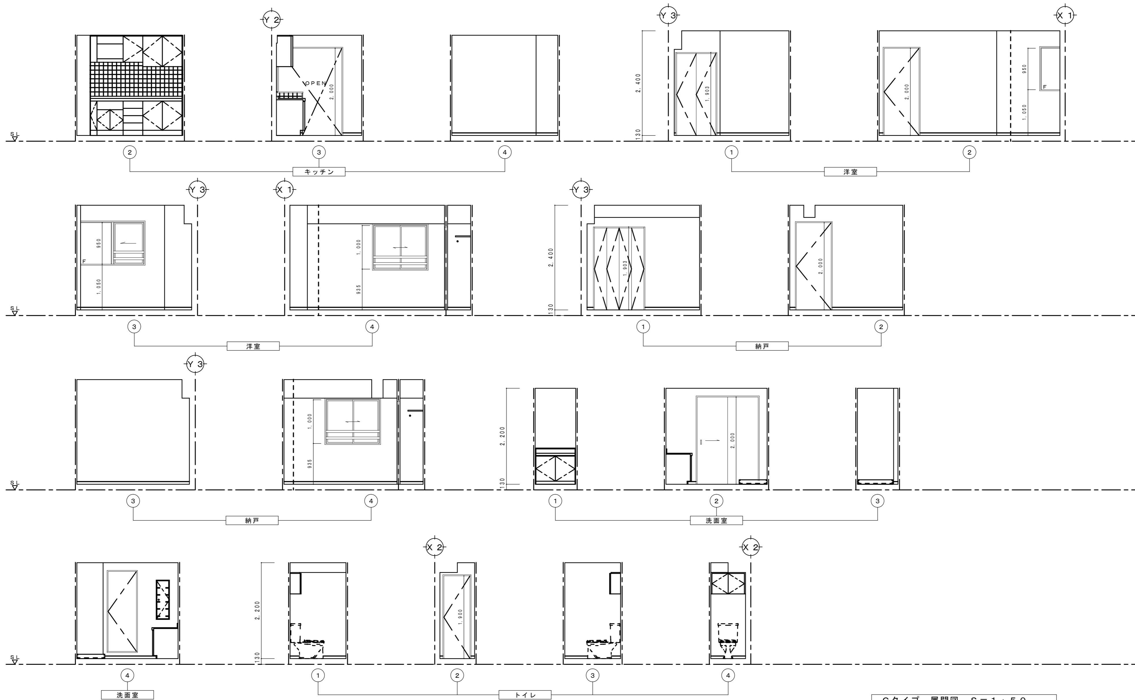
Cタイプ 展開図 S=1:50
